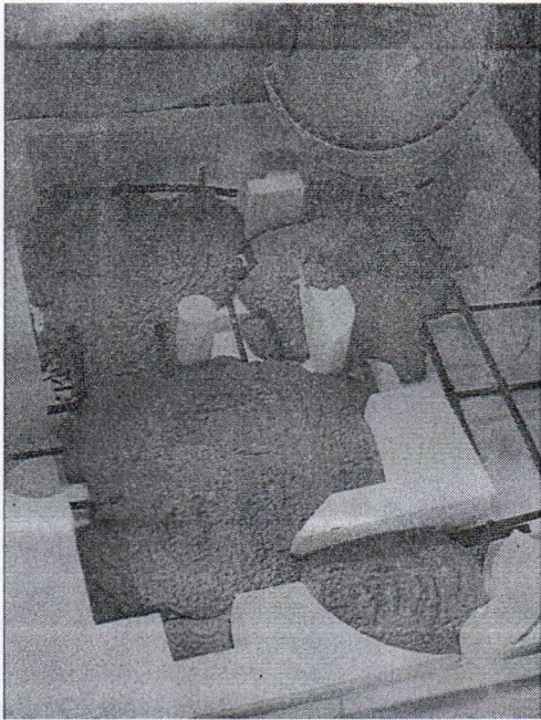
Proceso de fundición proyecto de escultura "Cimientos De Memoria"
