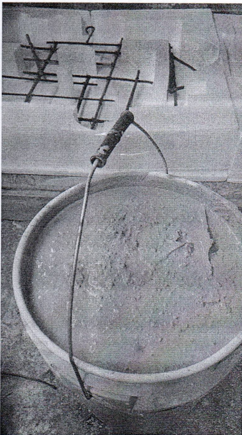
Armado de hierro, varillas de 1/2 y Concreto premezclado para la fundición
